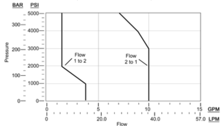
DTAF-*H* w/Bobine de haute puissance (Normalement ouvert)
