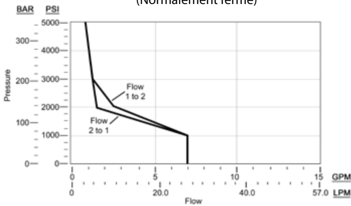
DTAF-*C* w/Bobine de faible puissance (Normalement fermé)
