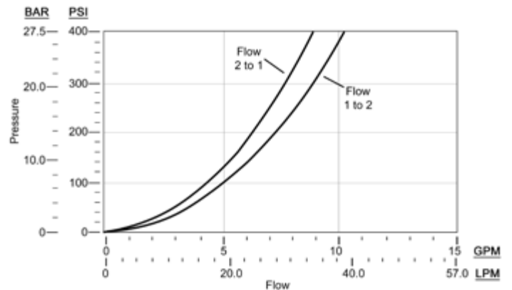
DTAF-*H* (Normalement ouvert)
