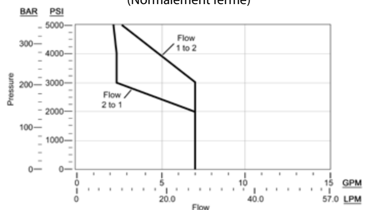
DTAF-*C* w/Bobine de haute puissance (Normalement fermé)
